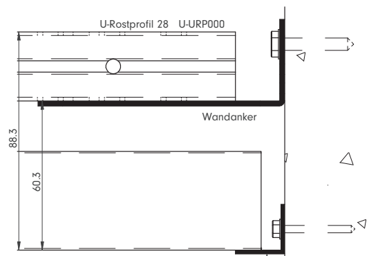
Einfachrandwinkel 20/20mm (RAL 9010) W-ERW020
